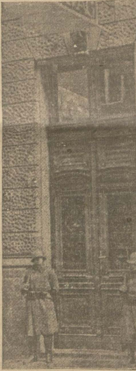
Viyana radyo merkezi zabitanın muhafazası altında
